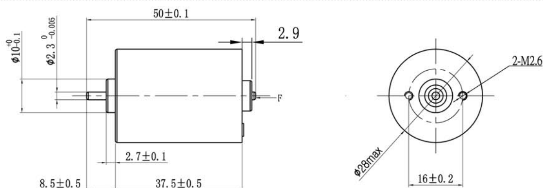
直流无刷电机 BLDC MOTOR
